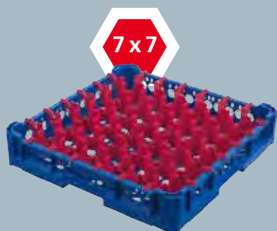
Cestello 50x50 cm con griglia rossa - 49 scomparti 50x50 cm rack with red divider insert - 49 compartments
